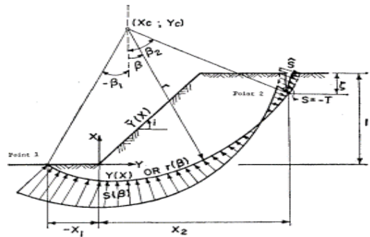
Gambar 2 Tension cracks pada lereng (Baker, 1981)
