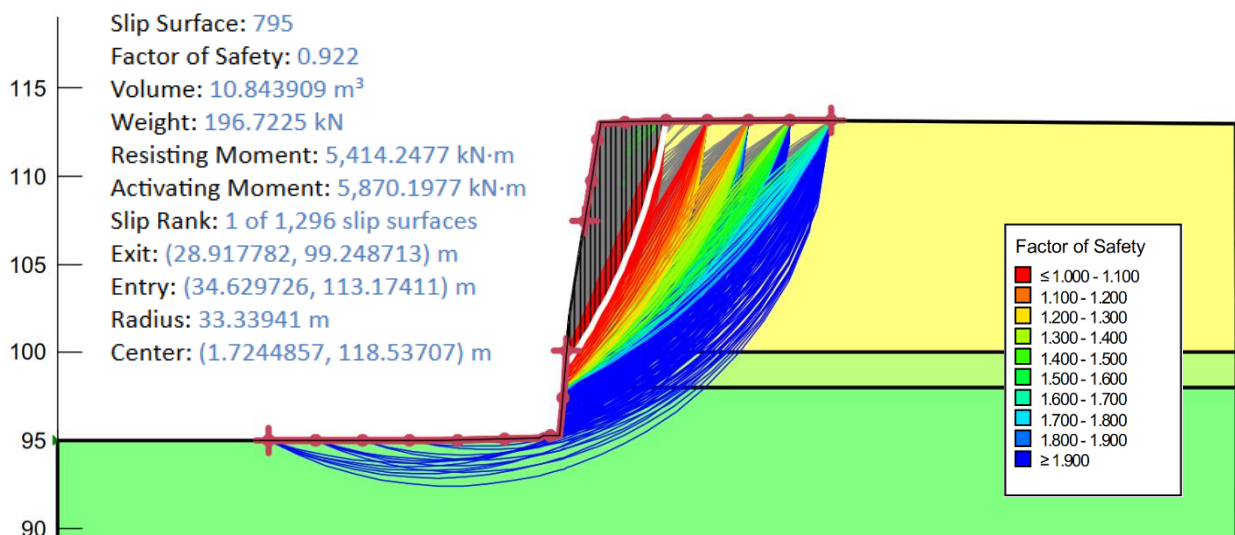
Gambar 4 Pemodelan tebing kondisi natural slopes
