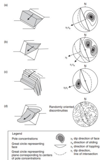
Gambar 1. Tipikal keruntuhan batuan (a) planar; (b) wedge; (c) topples; (d) circular (Wyllie & Mah, 2004)
